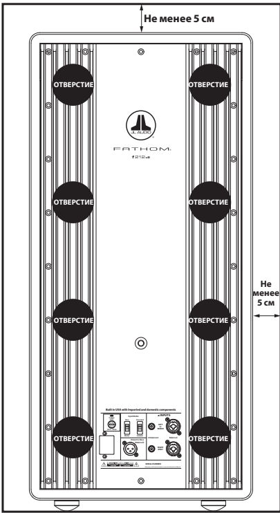
Вид сзади на установленный корпус (f212):
