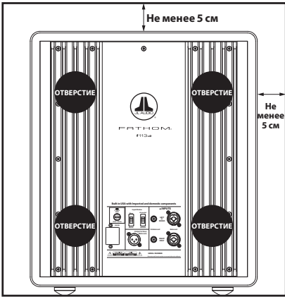
Вид сзади на установленный корпус (f110, f112, f113):
