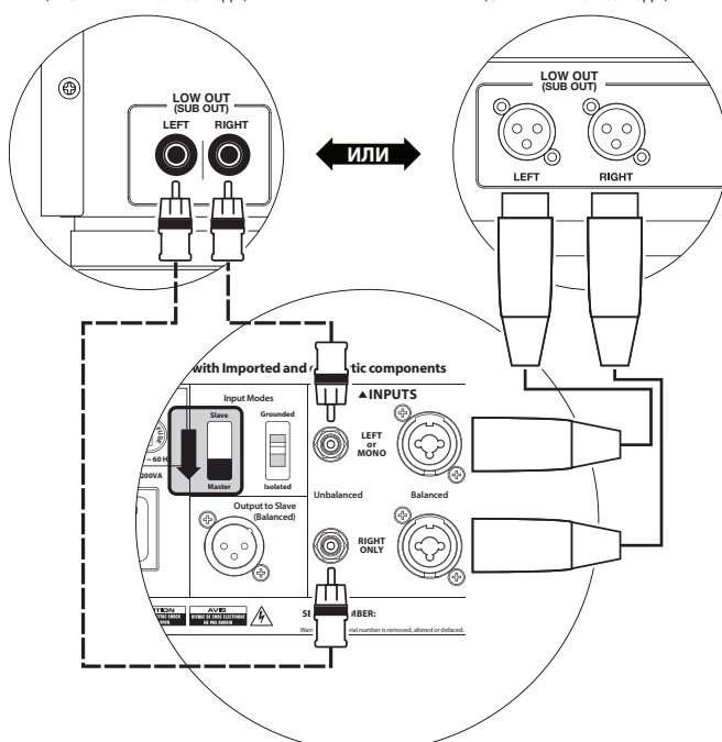
ЭЛЕМЕНТЫ УПРАВЛЕНИЯ НА ЗАДНЕЙ ПАНЕЛИ САБВУФЕРА FATHOM (ВЕДУЩЕГО)
